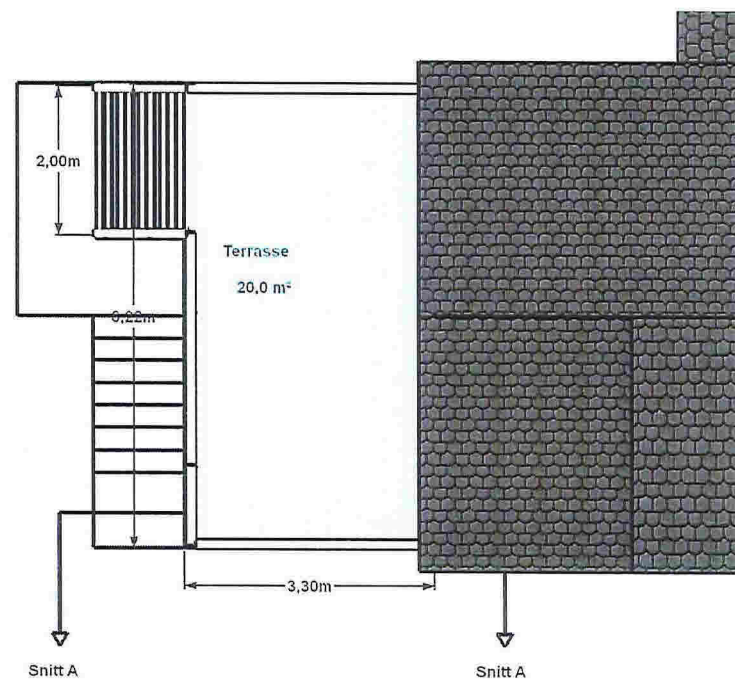
Snitt A
