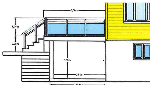
Snitt A-A
