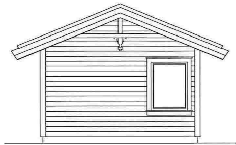
FASADE NORD
