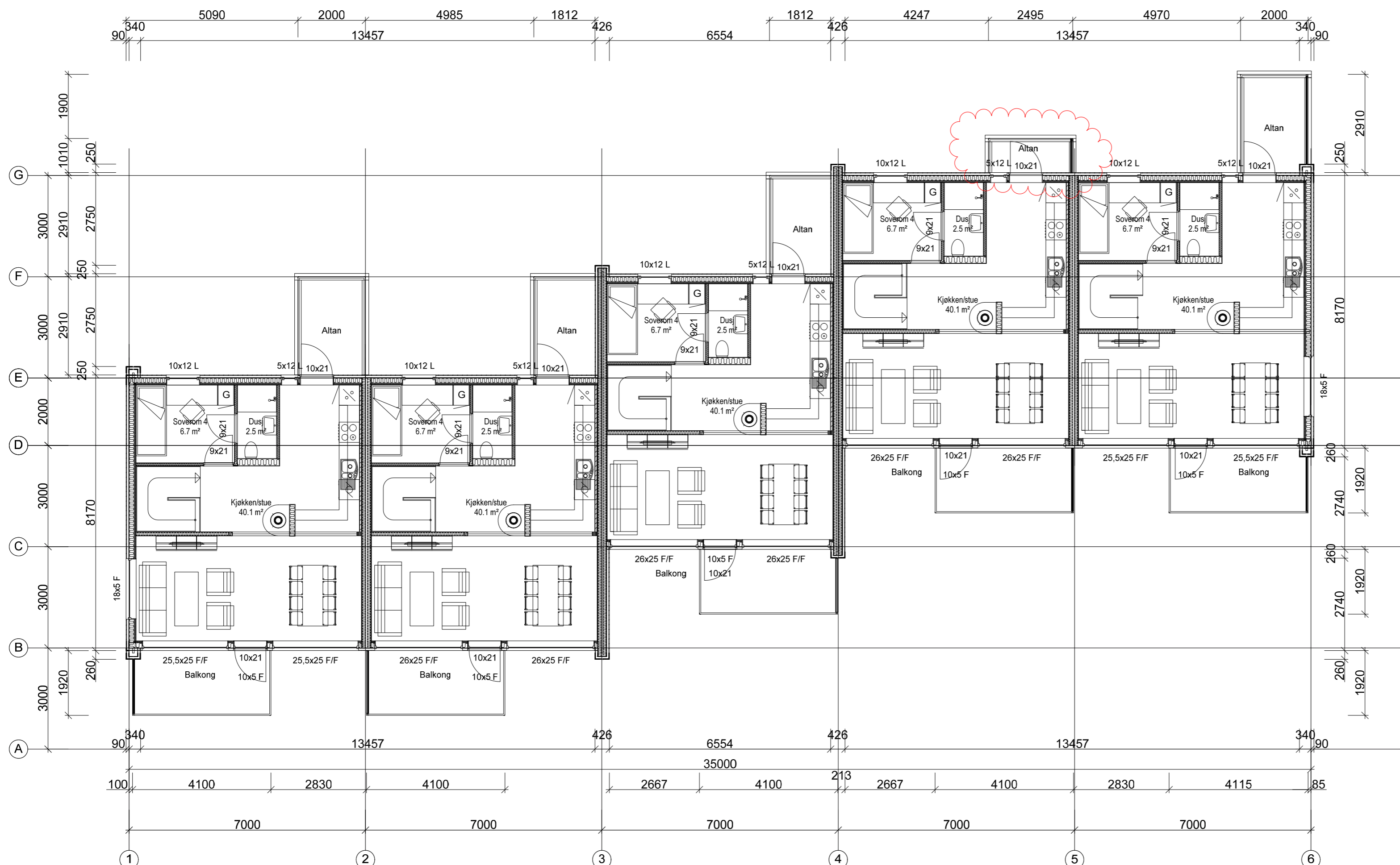
BOLIG 30 Plan 2. etasje BRA 50,1 m 2
