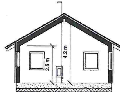
Snitt B-B
