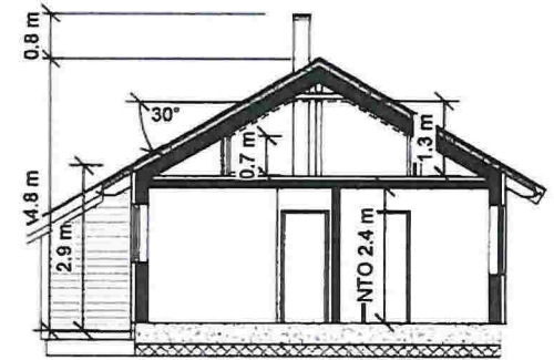
Snitt A-A
