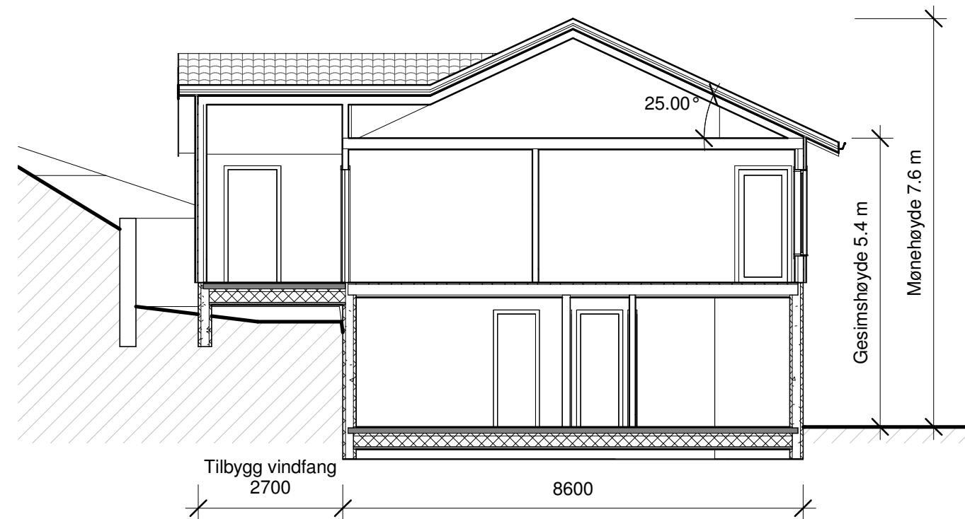
2 Snitt B-B 1 : 100
