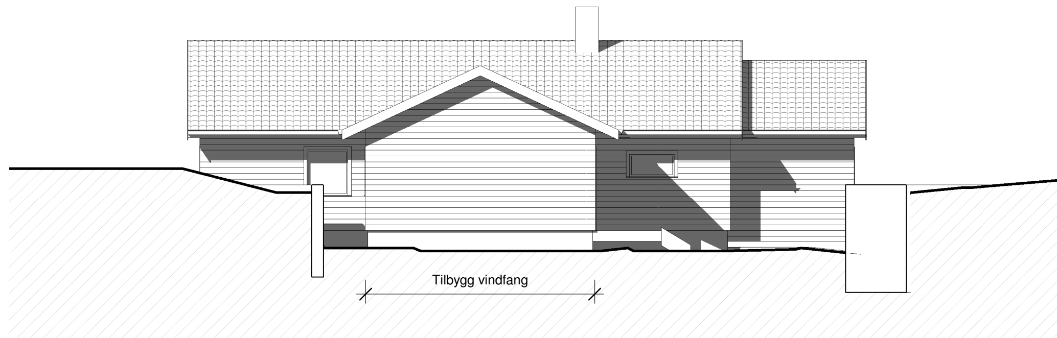
1 Øst 1 : 100
