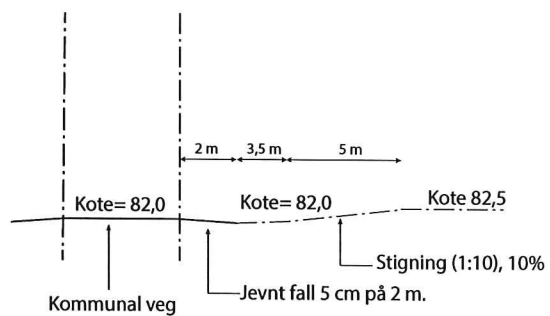
Profil A-A
