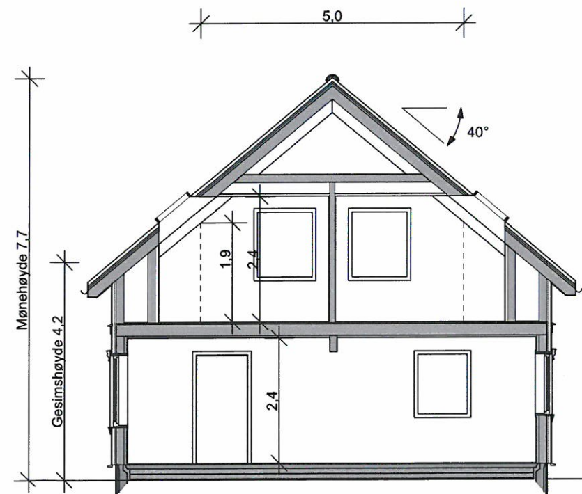
SNITT A-A
