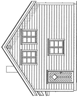
FASADE NORD
