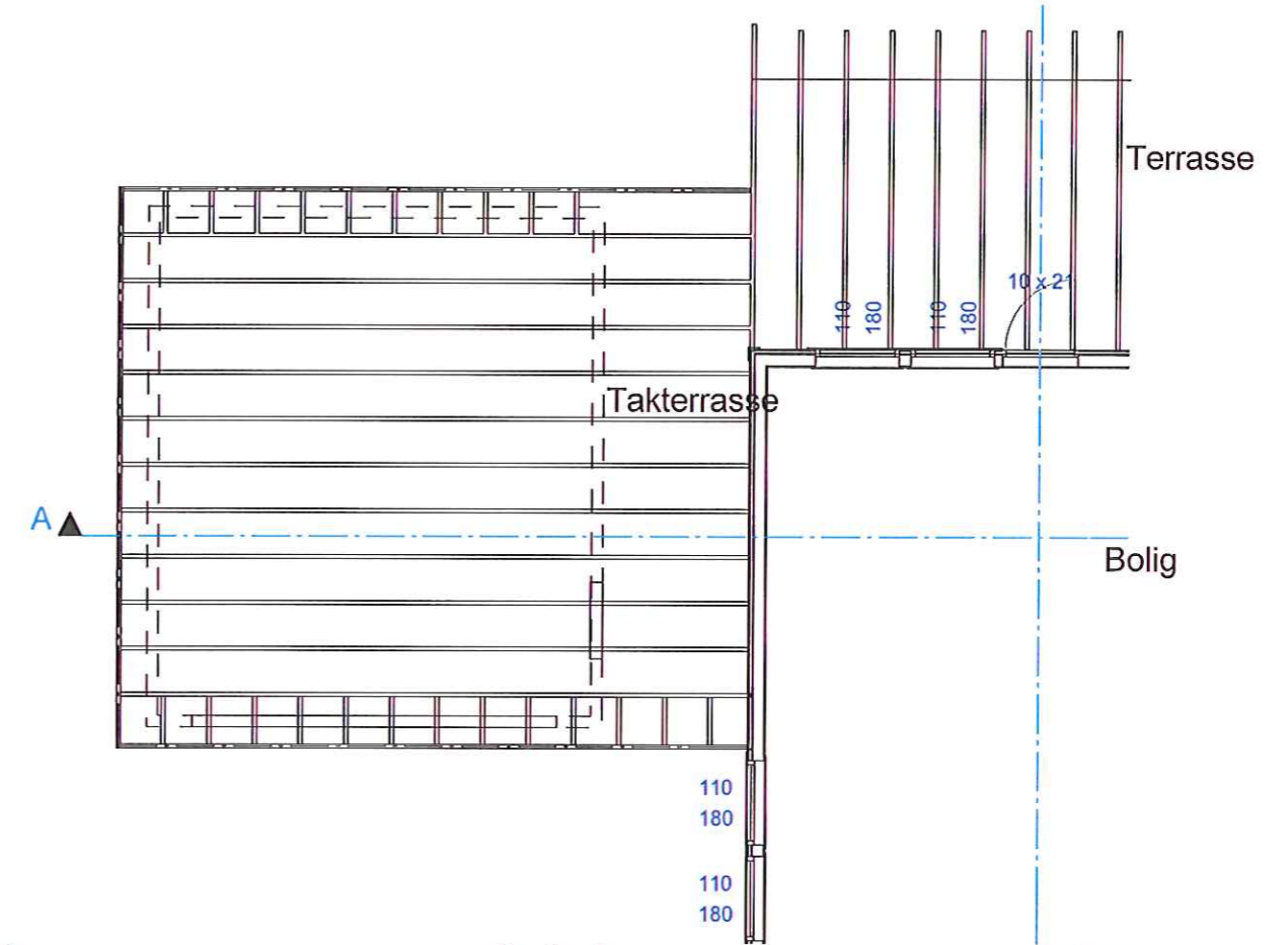
1. 2. etasje 1:100
