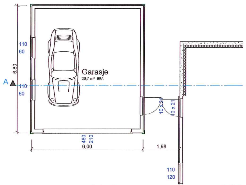
0. 1. etasje 1:100
