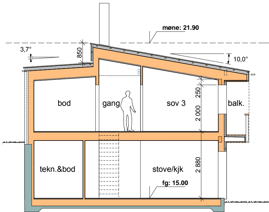
Snitt A-A
