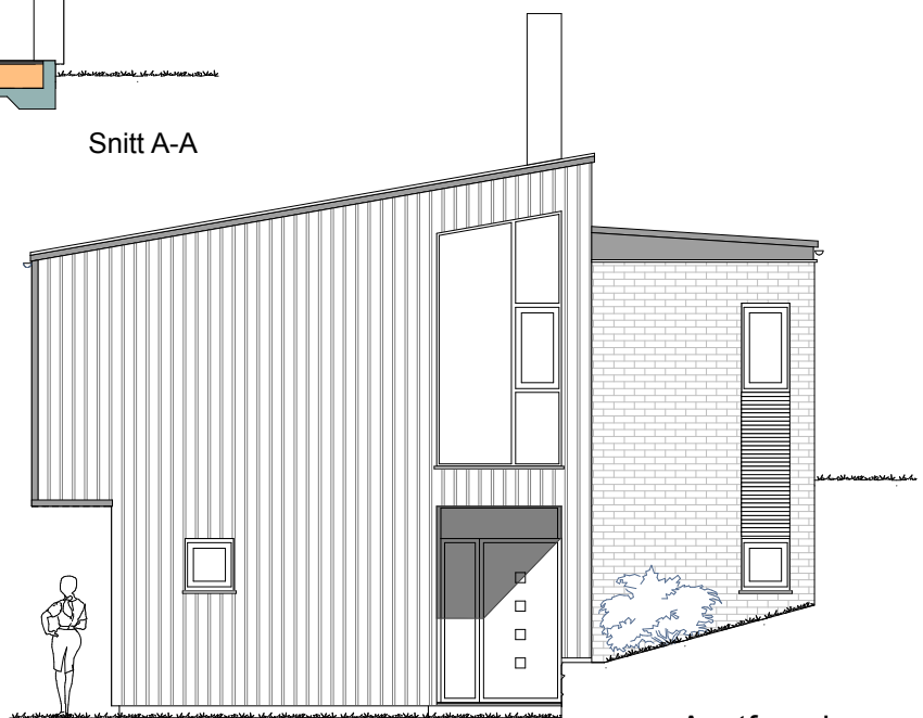
Ausfasade
