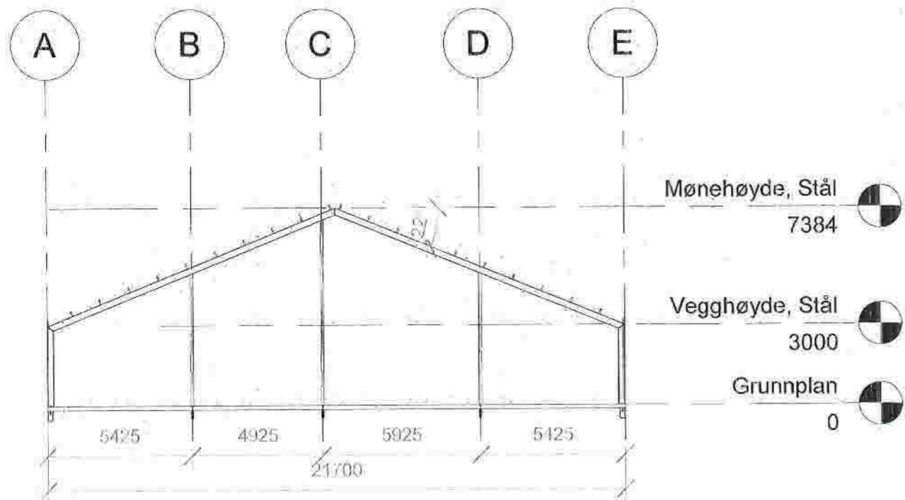
1 Akse 1 1 : 200
