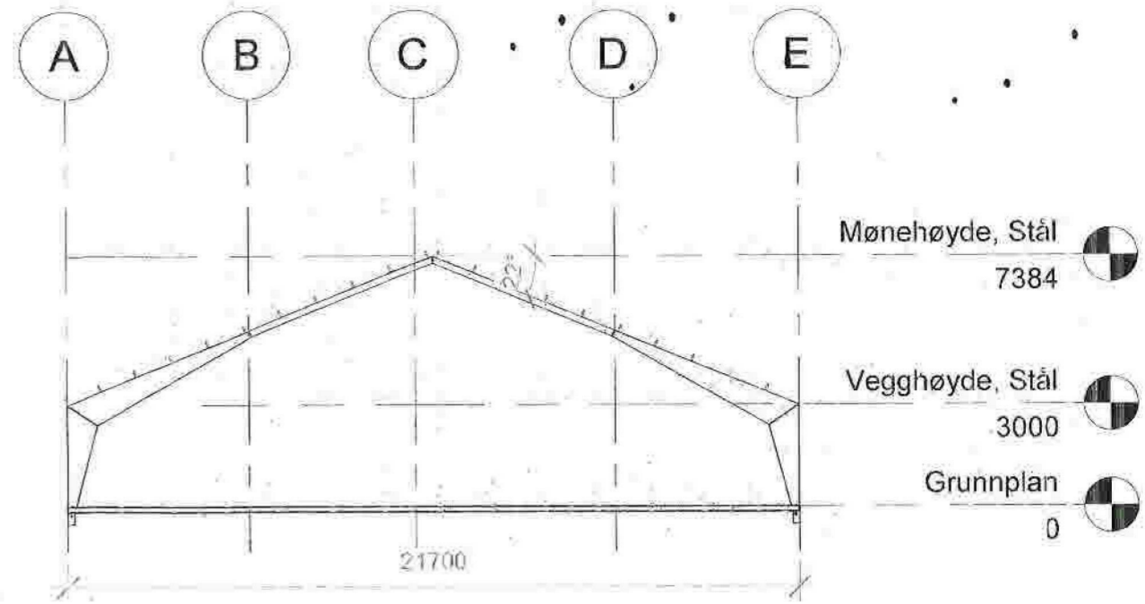
2 Akse 2-5 1 : 200
