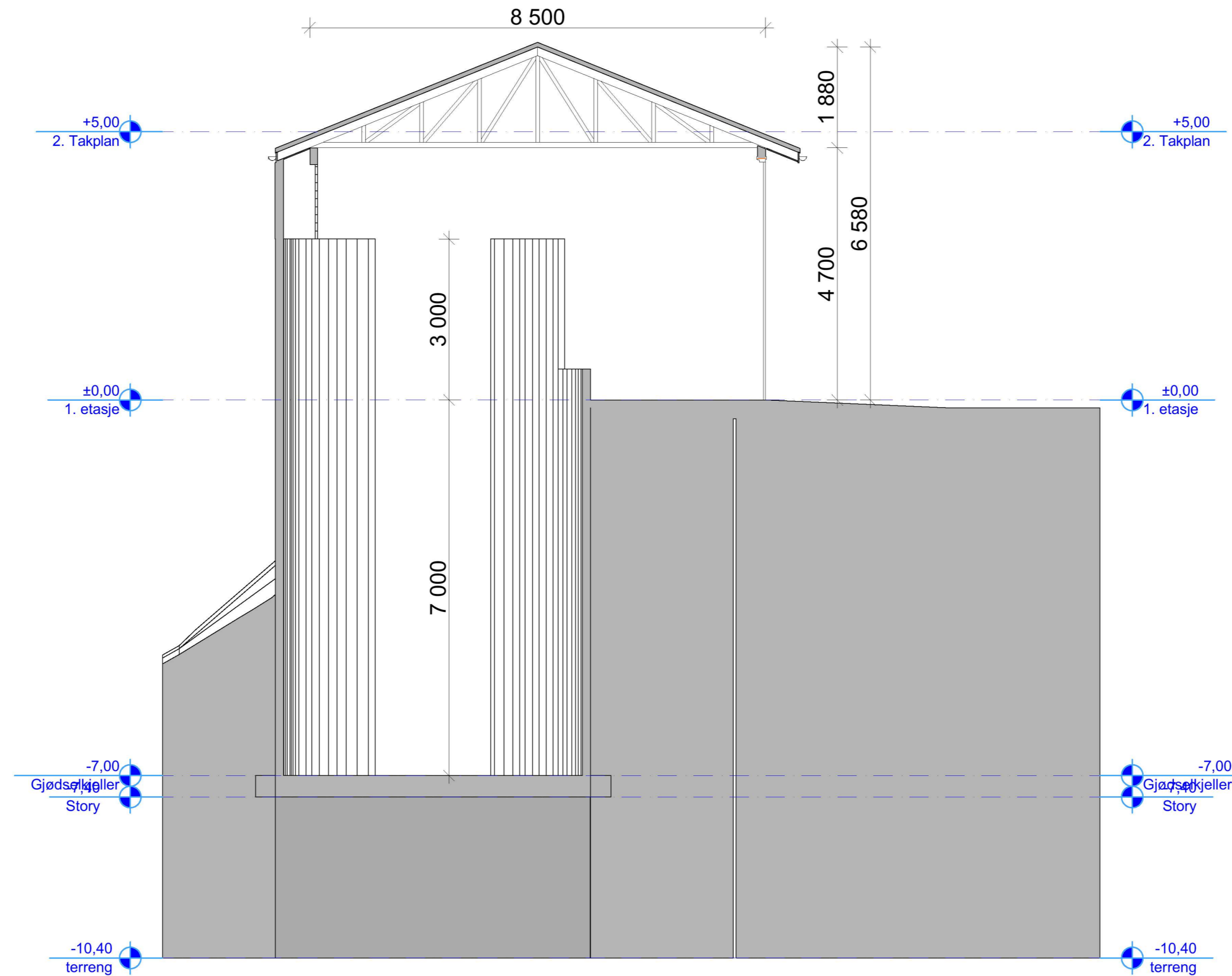
1:75 Snitt A
