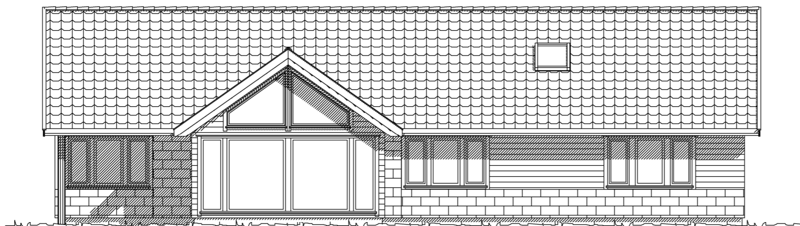
FASADE SØR
