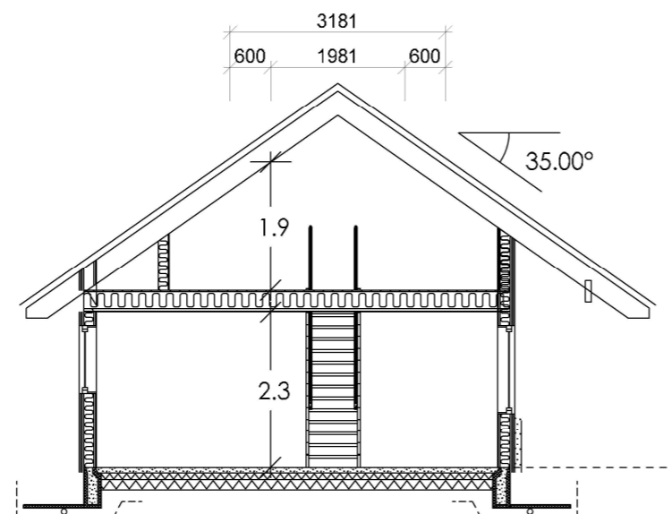
Snitt B-B
