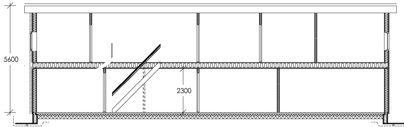
Snitt A-A
