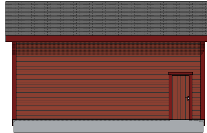
LANGVEGG TYPE 2
