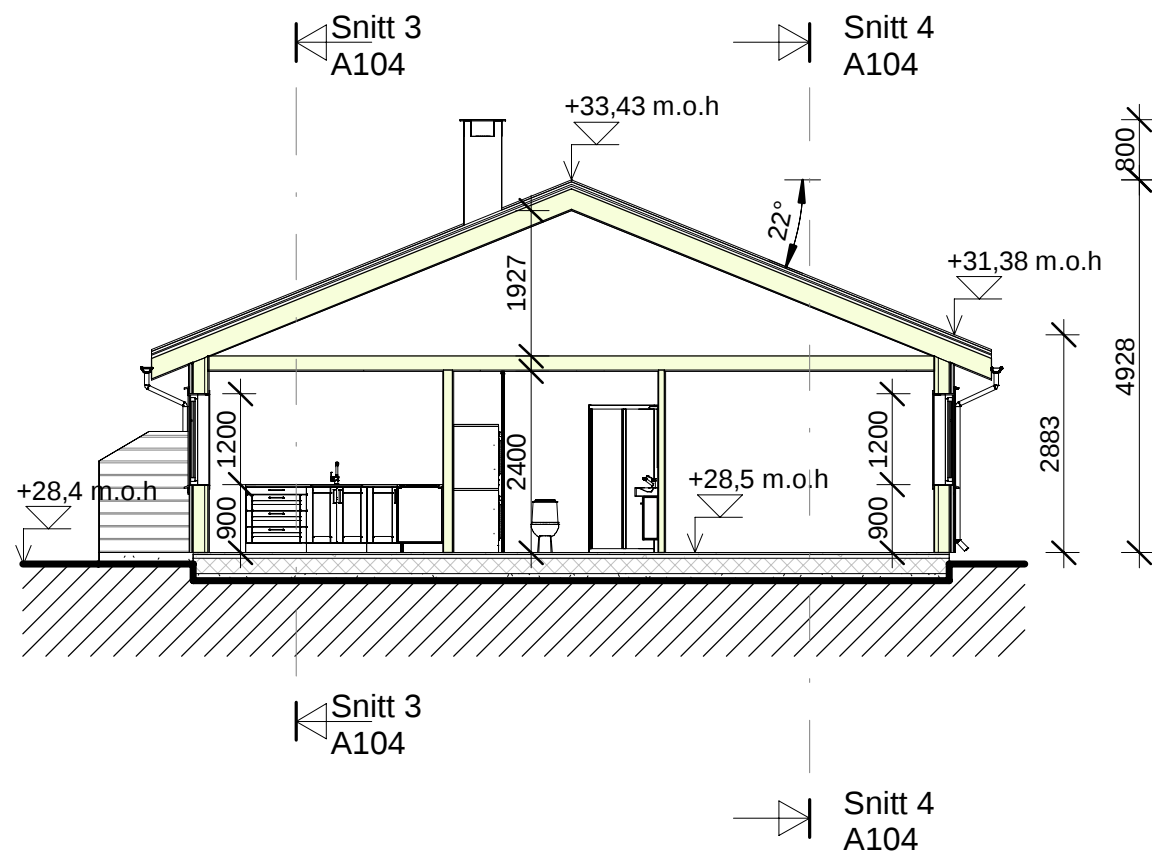
Snitt 1 1 : 100
