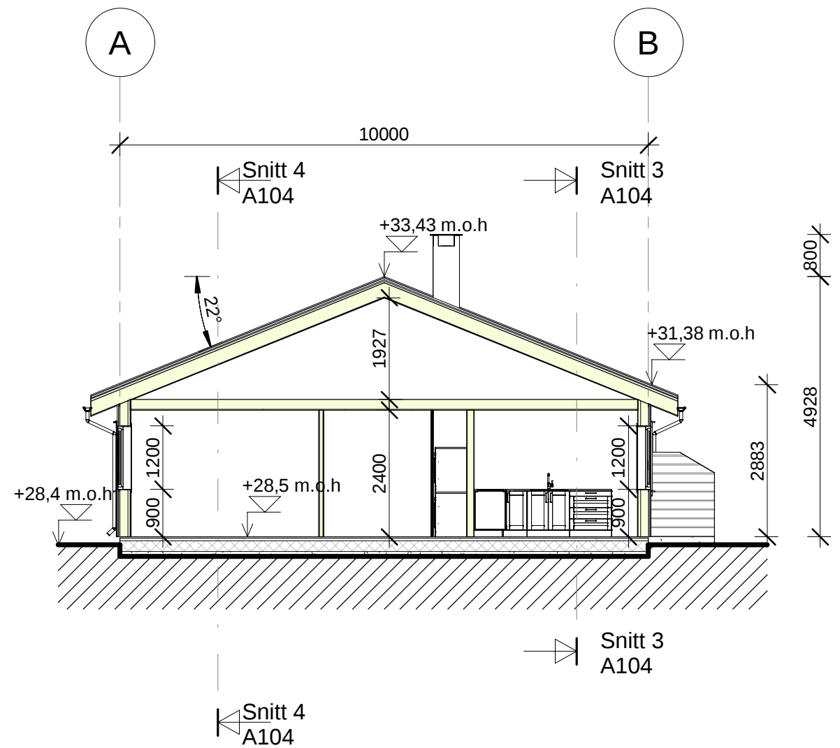
Snitt 2 1 : 100
