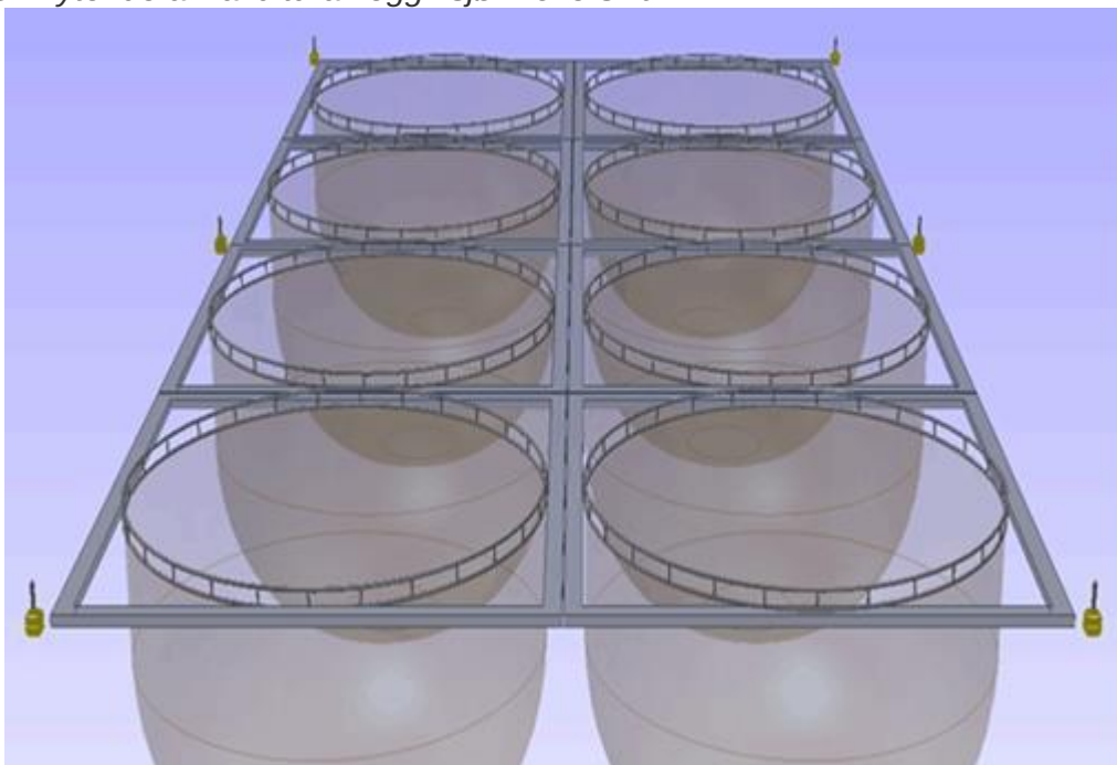
Figur 3. Flytende akvakulturanlegg i sjø – oversikt
