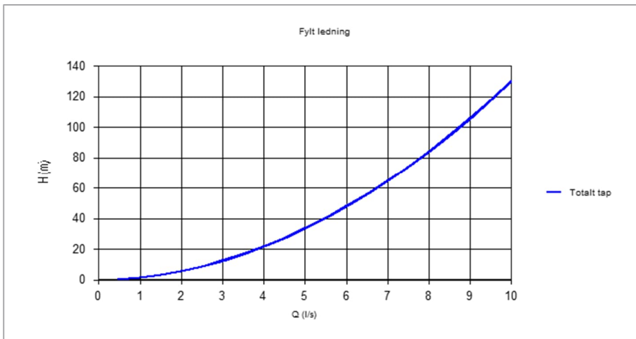
Figur 18: Trykktap i eksisterende sjøledning mellom Hosteland, Straumsvika og Haugsdal (kjelde: Cowi)
