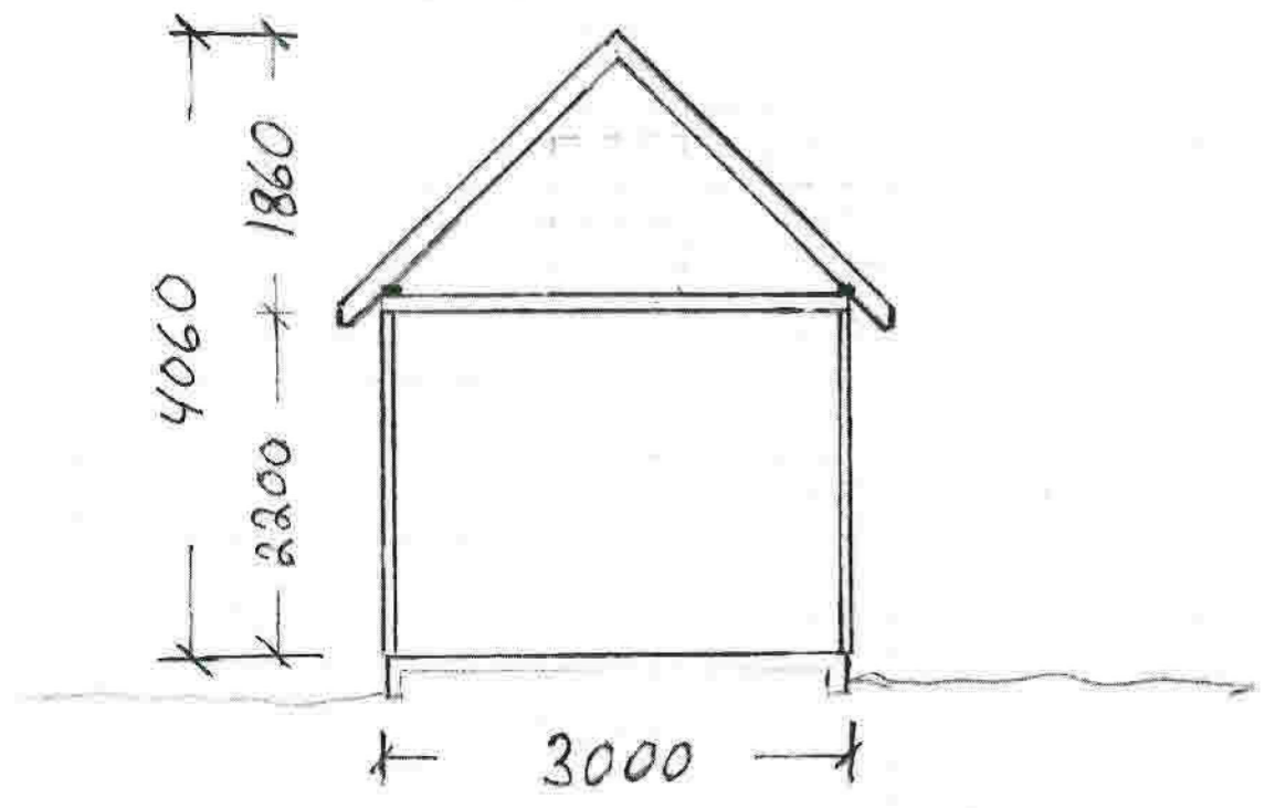
Snitt 1:50
