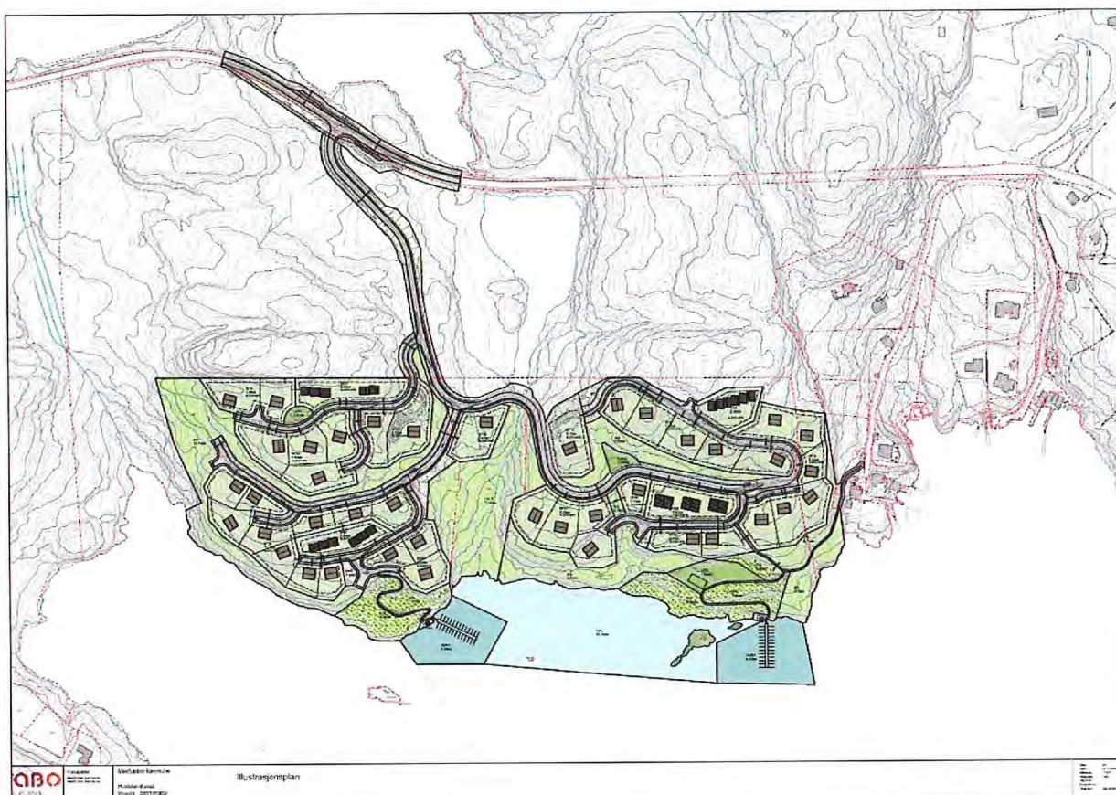
Figur 1. Illustrasjonsplan.
