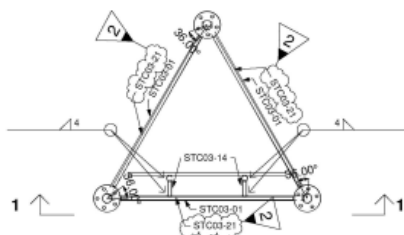
Snitt 2-2 1 : 20
