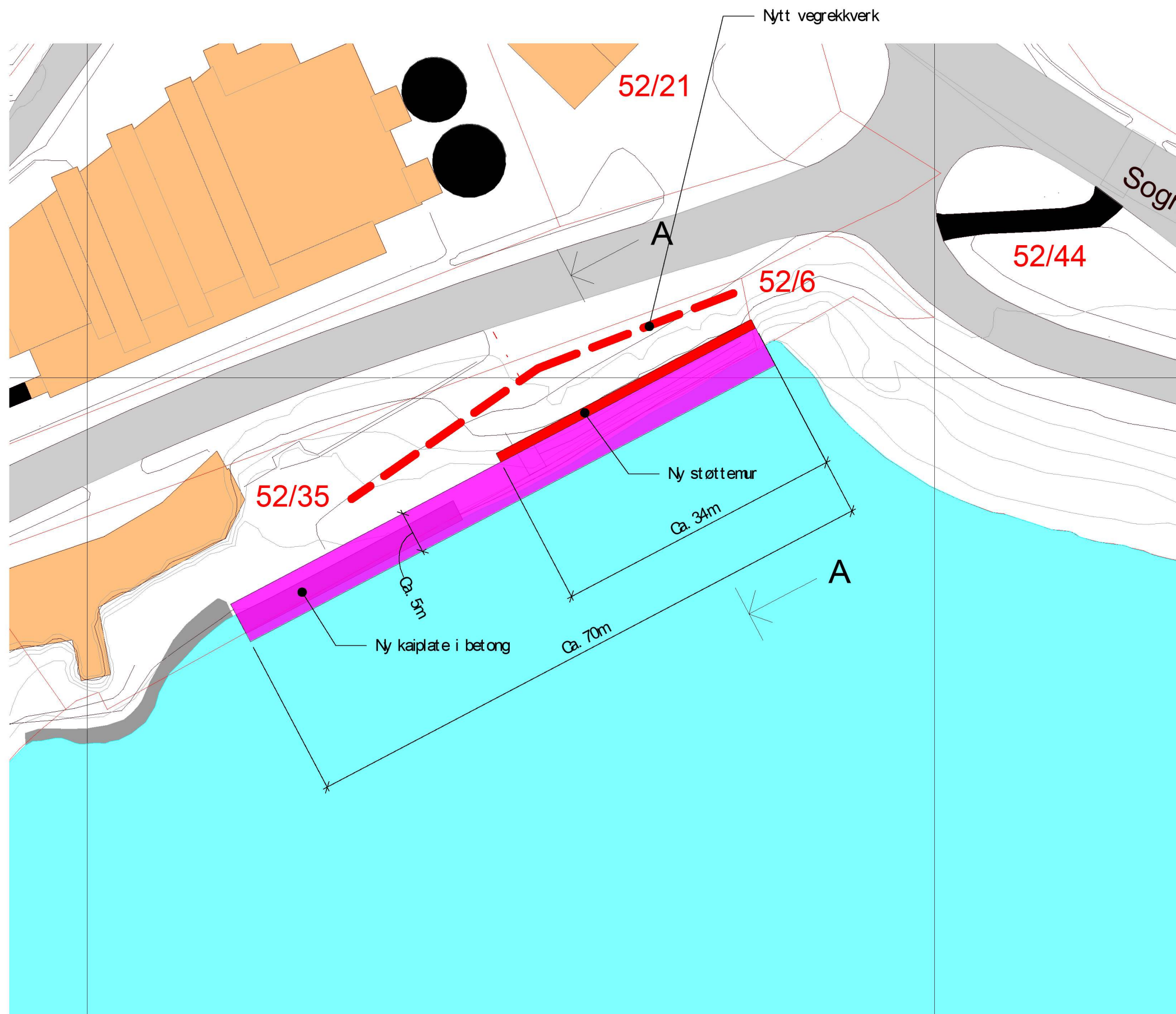
Kartutsnitt. Plan. Kai i Matre 1 : 500
