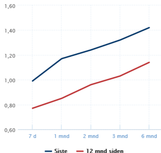
Nibor rentekurve
