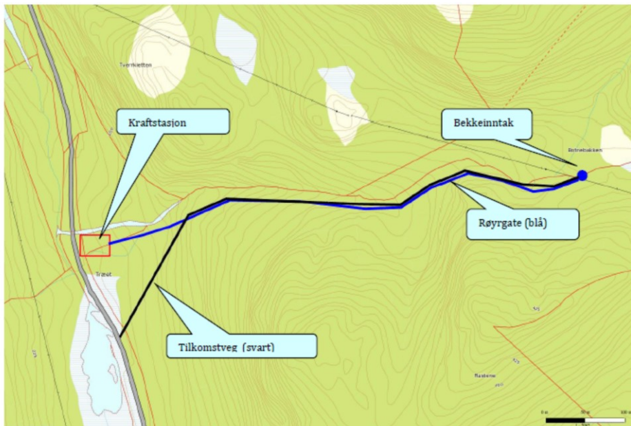
Figur 3. Kartutsnittet viser i grove trekk dei viktigaste naturinngrepa i form av inntak, rørgater (blå), veg (svart) og kraftstasjon.
