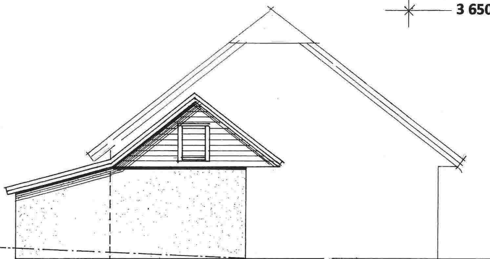
Fasade mot NØ
