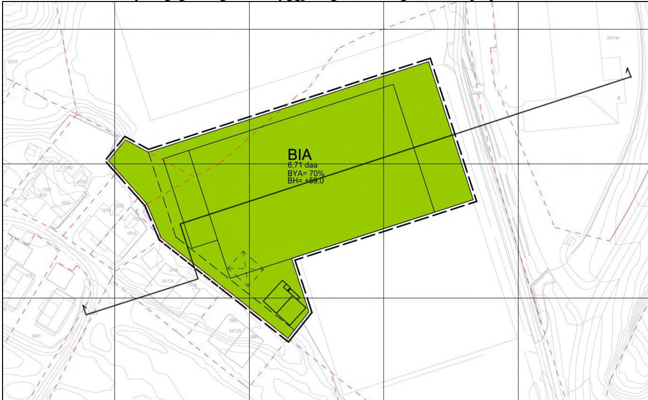
Figur 22 Framlegg til detaljplan, illustrasjon med planlagd hall og terrengprofil A
