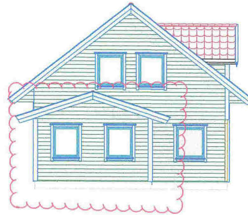
Fasade Øst
