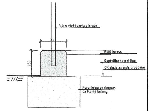
Snitt 1-1 1:10
