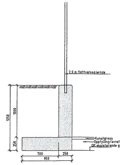
Snitt 2-2 1:20
