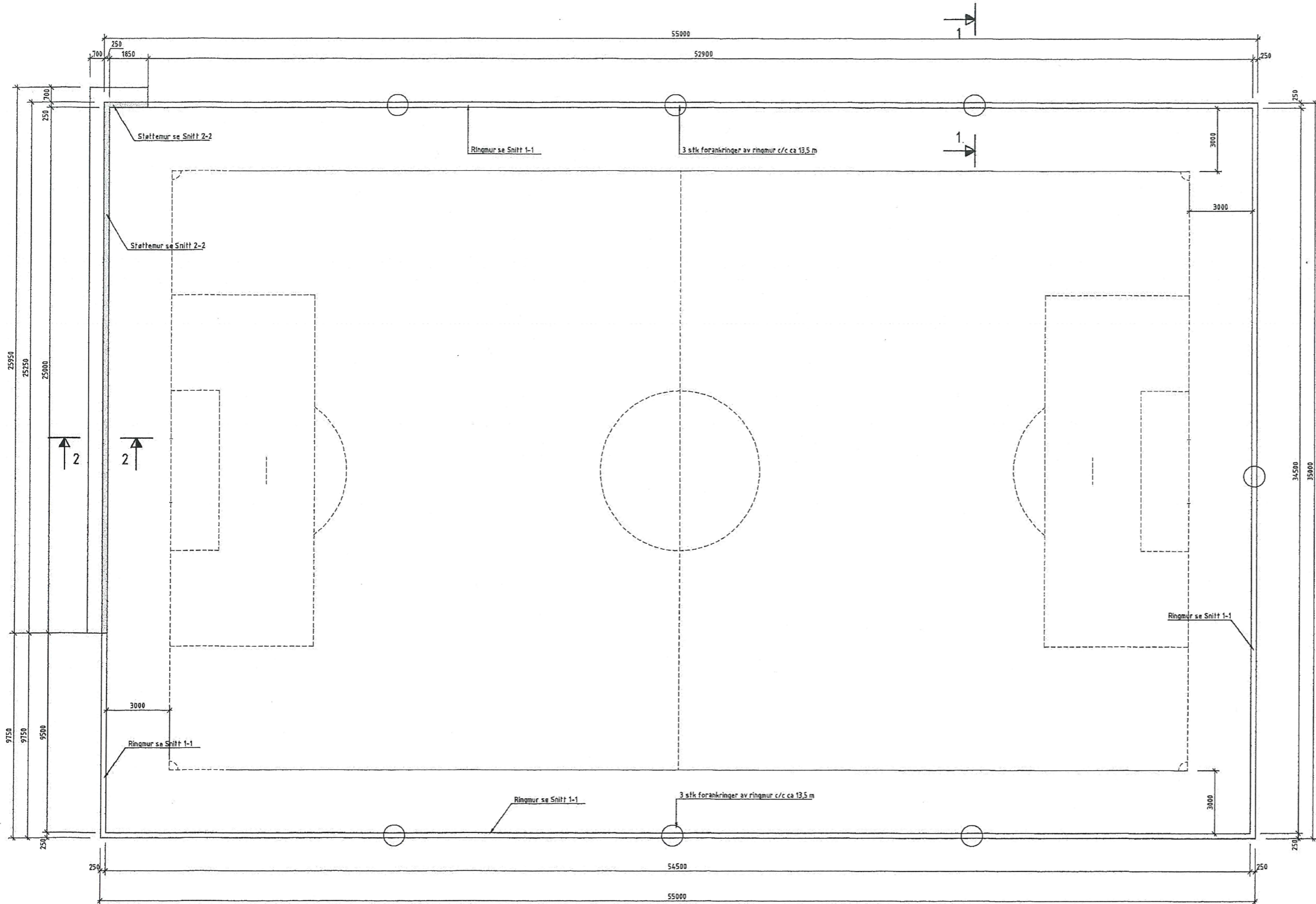
Plan 1:100
