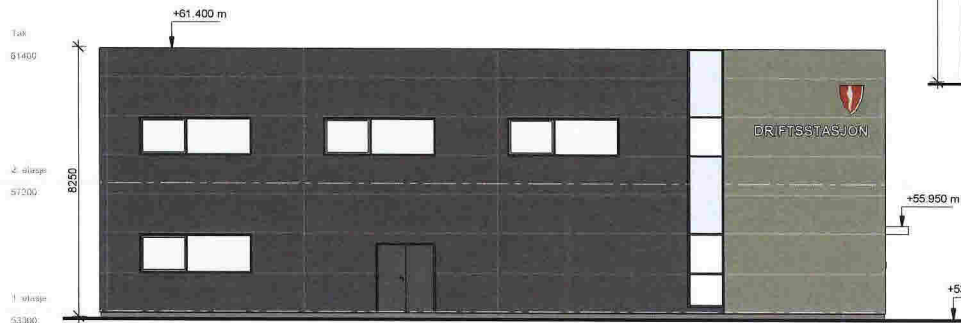
1 Fasade mot nord-øst 1: 100
