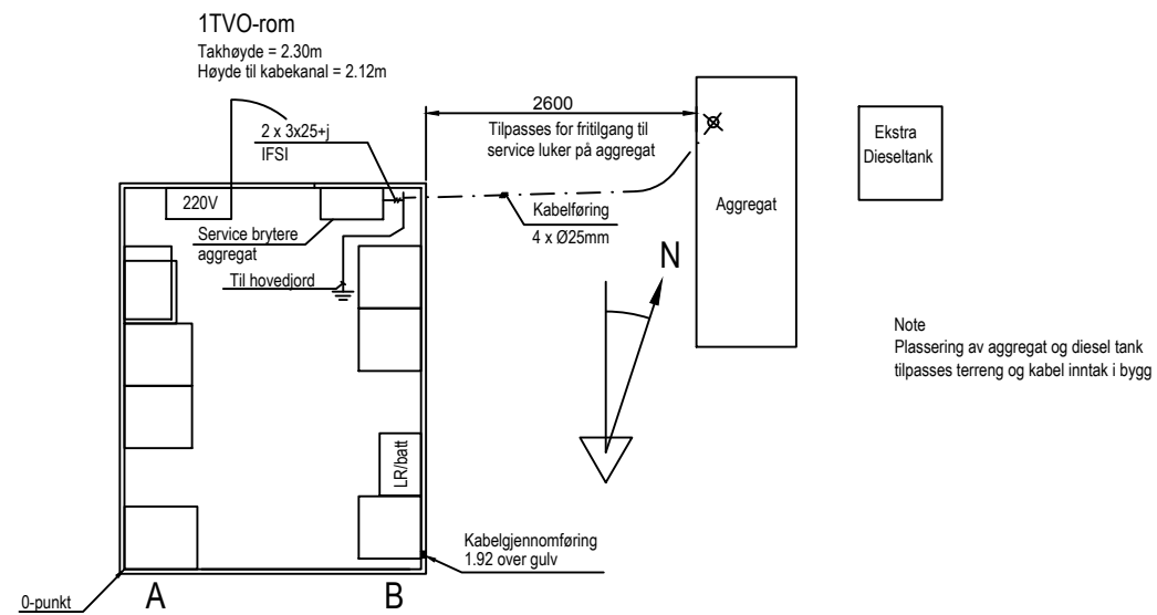
Utstyrsplassing / orienteringsplan M 1 : 50
