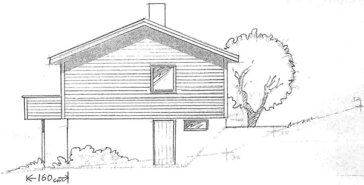
FASADE MOT NORD M 1:100
