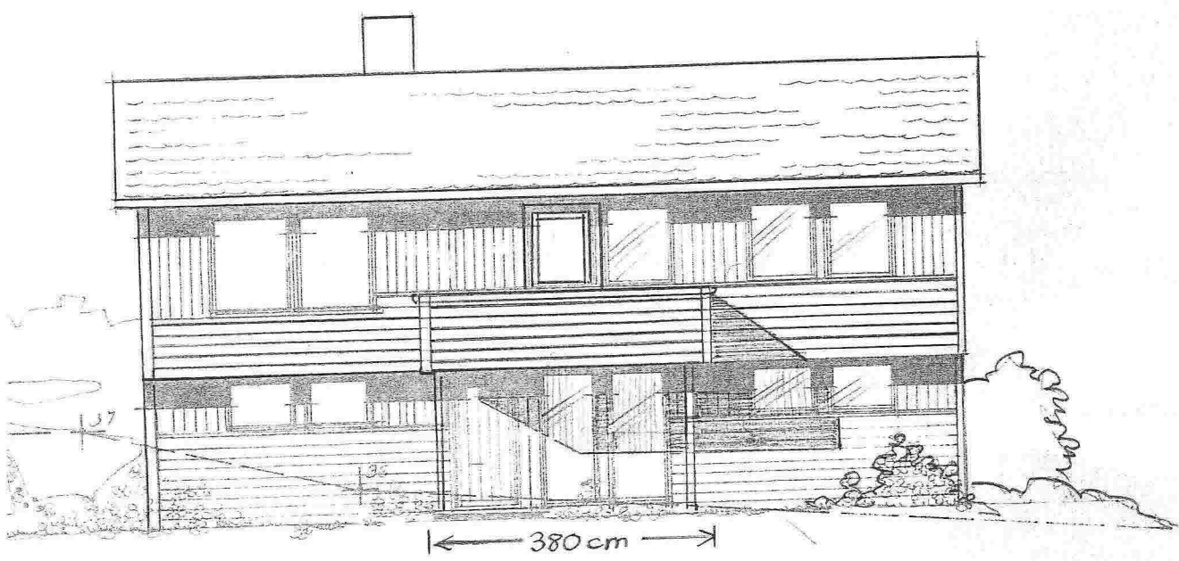
FASADE MOT ØST M 1:100
