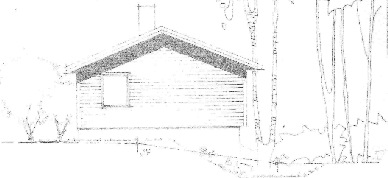
FASADE MOT SUD
