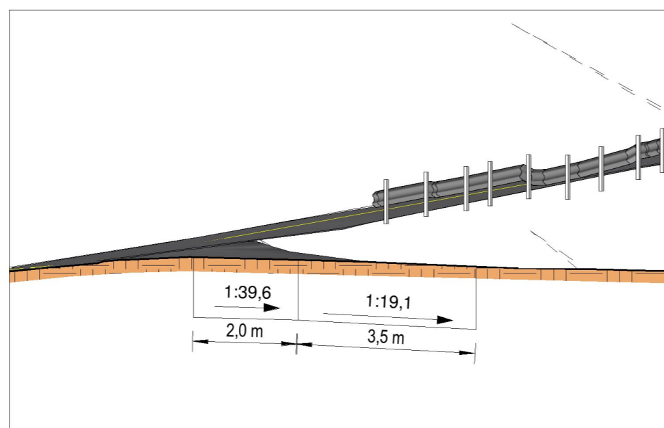
Lengdeprofil 1 : 100
