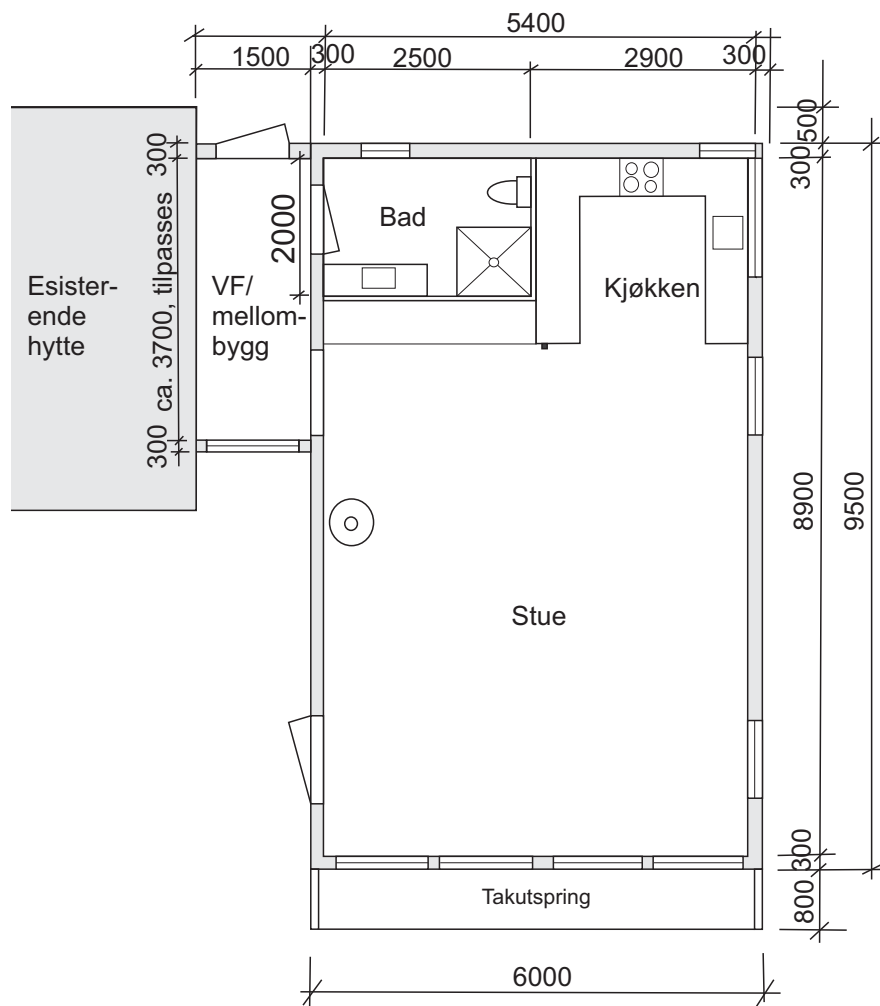
Plan tilbygg
