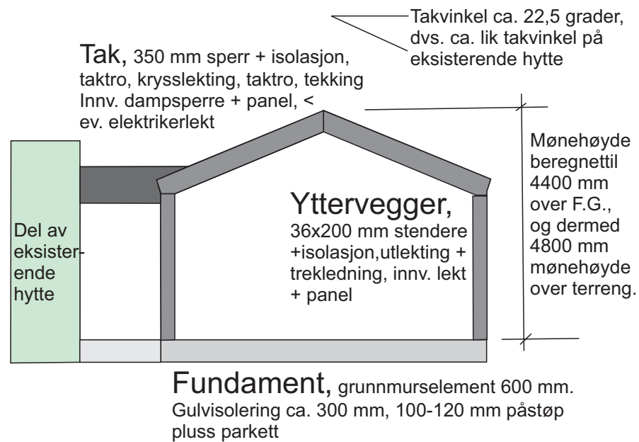
Snitt, tilbygg
