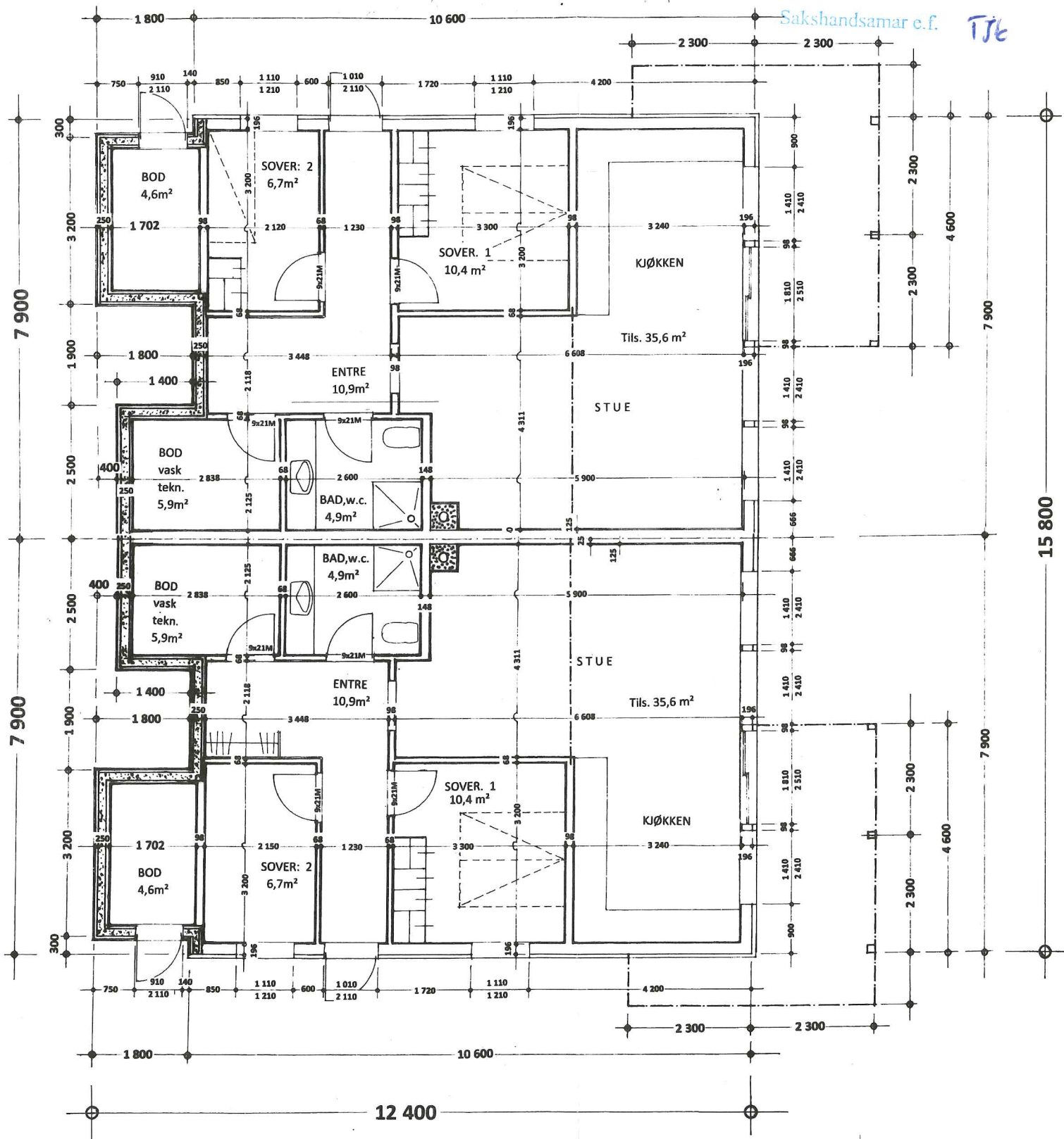
PLAN underetasje
