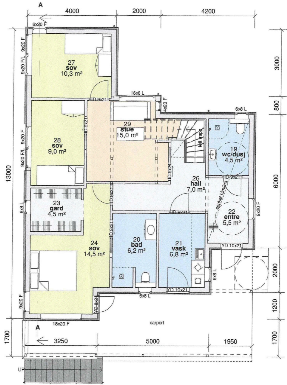
1. Etasje 1 : 100
