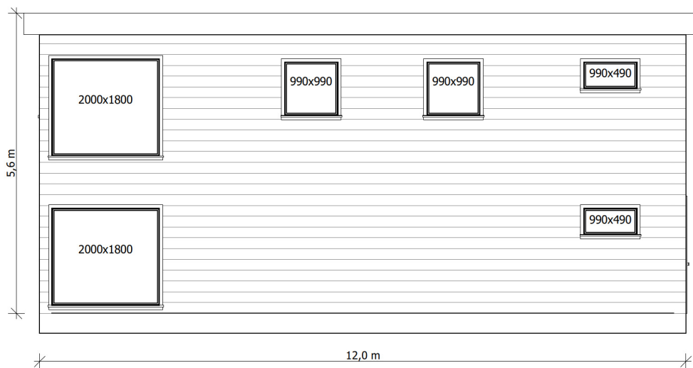
C Fasade 3 1 : 100
