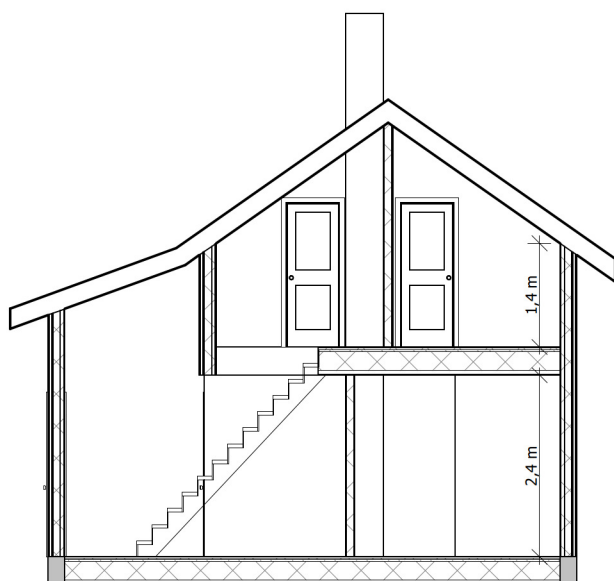
E Snitt 1 1 : 100
