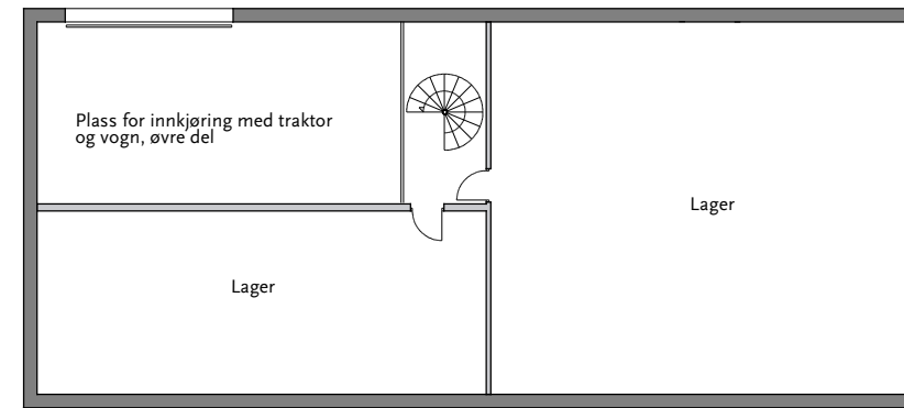
Plan loft
