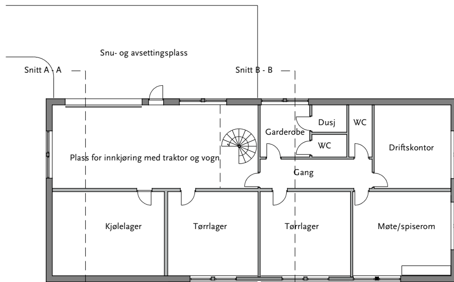
2 etg. 324 m 2
