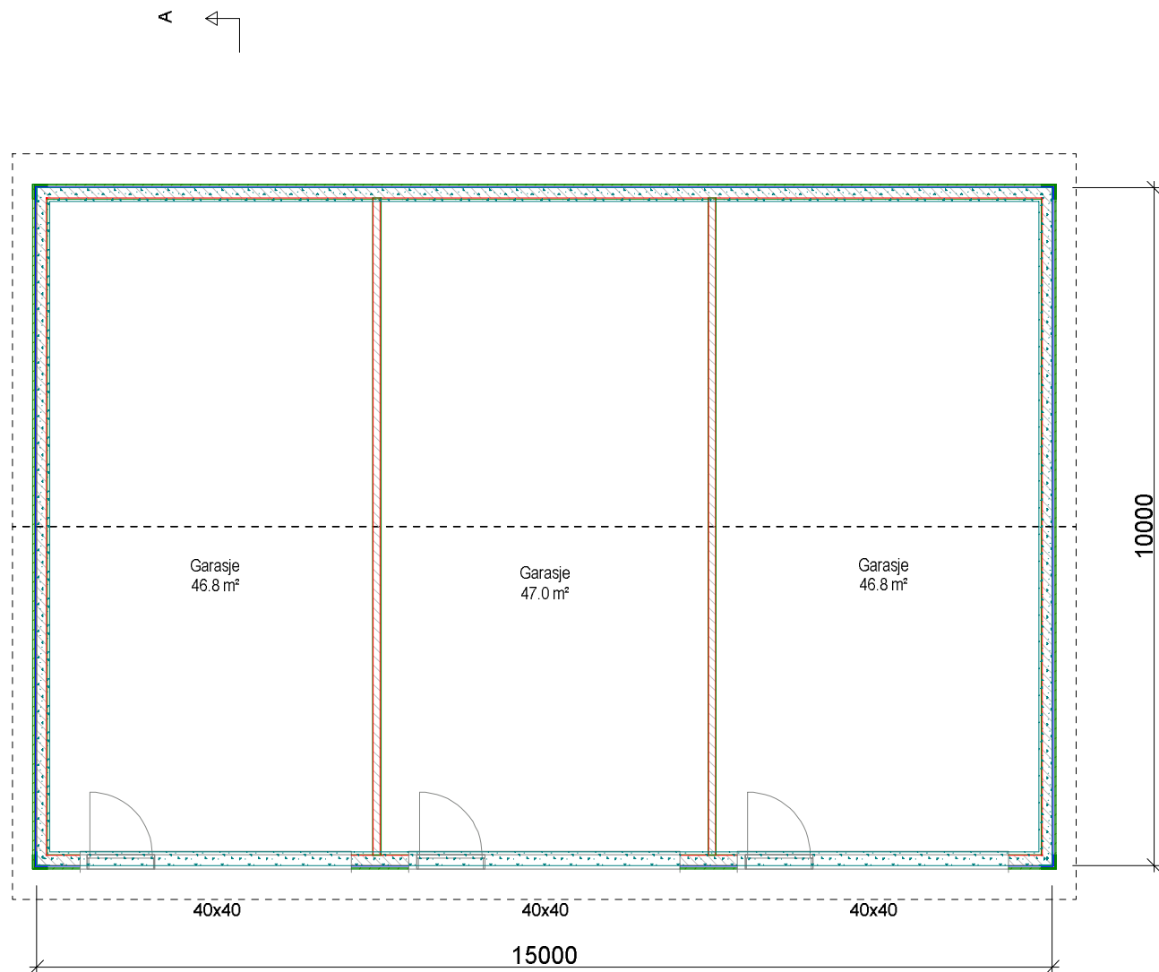
PLAN GARASJE
