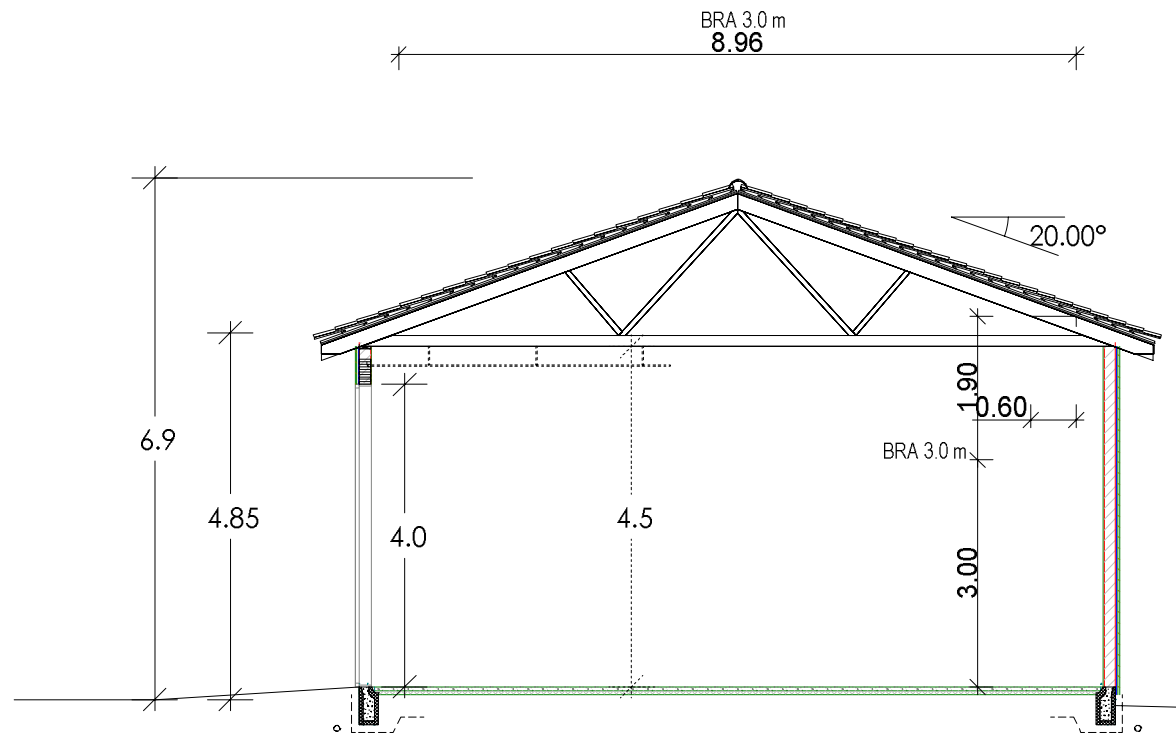
SNITT A-A
