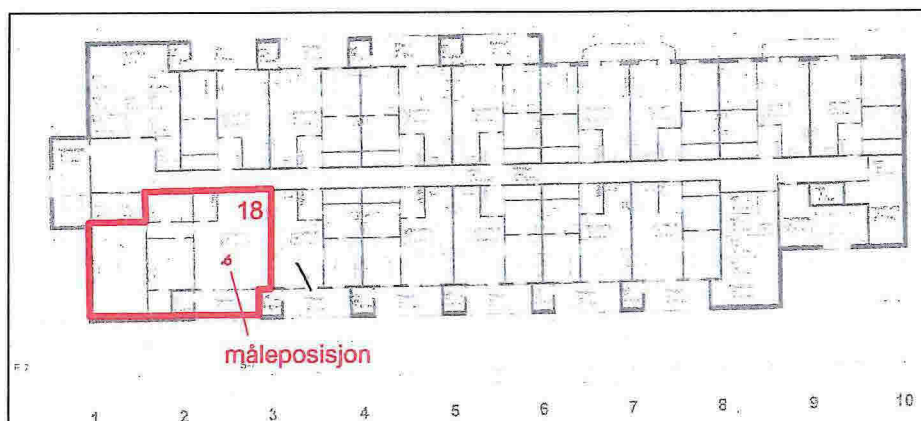
Figur 3 – Plantegning 3. etasje, Sameiet Frekhaug Senter, inkl. måleposisjon i stuen til leilighet 18
