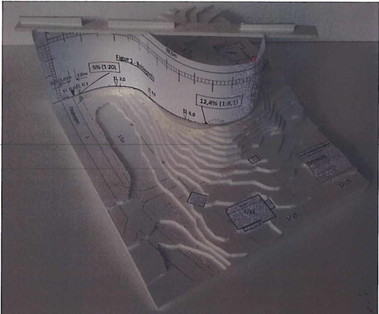
Figur 1: Skalamodell som illustrerer bakke profil maksimum 12,4% stigning
