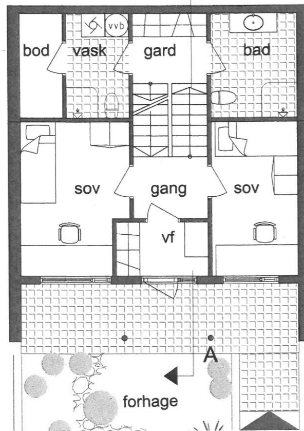
u.etasje
