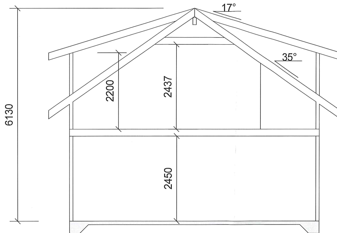
SNITT A-A
