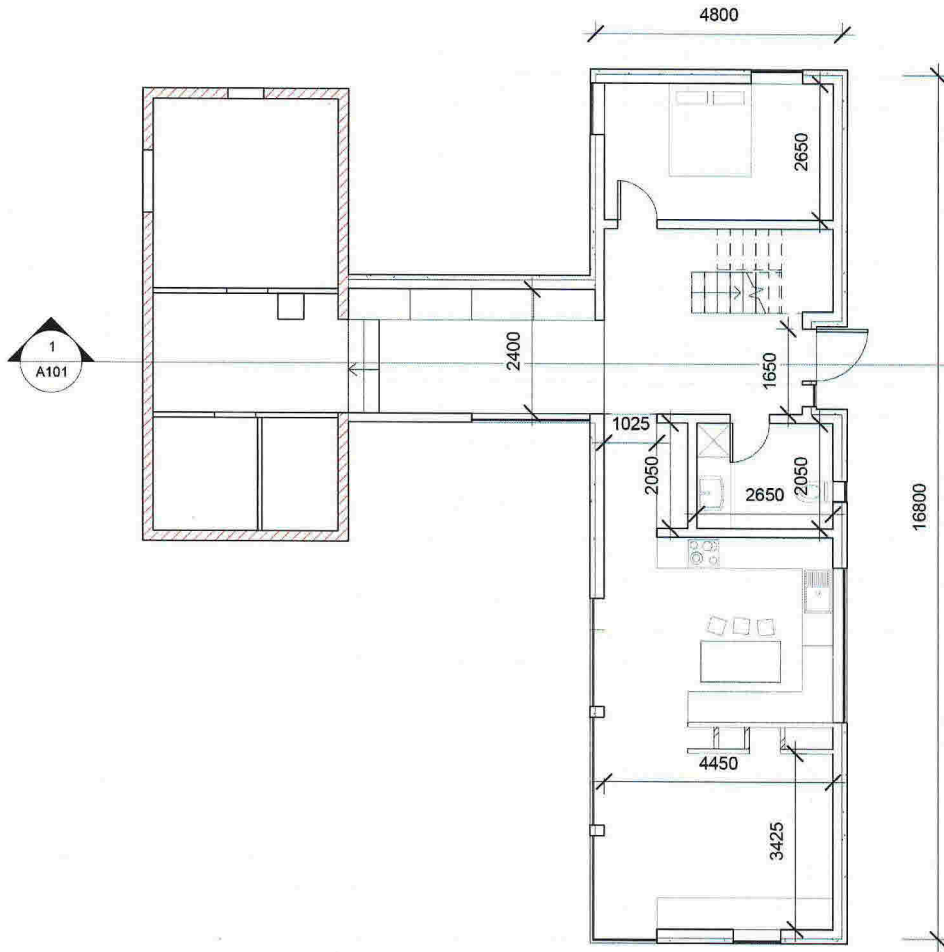
Plan 1. etg 1:100
