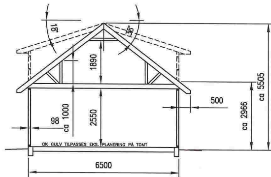
TYPISK SNITT
