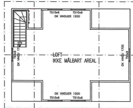
LOFTSPLAN
