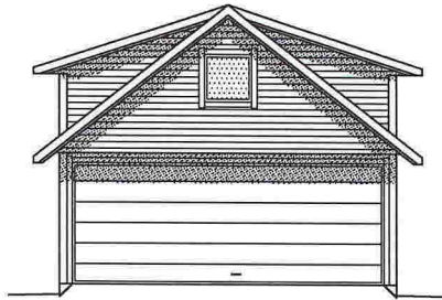
FASADE NORD
