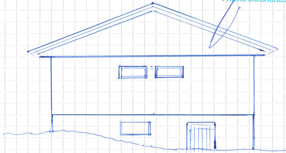
Fasade mot øst ( 1 : 100 )
