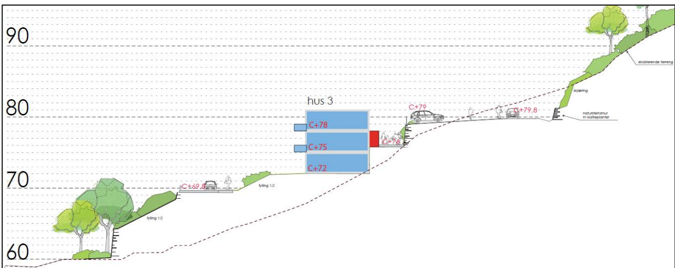
Figur 23. Snitt 4 viser området BKS2 med løsning for tilkomst til bustadane, gatetun og parkering i terrenget (ABO Plan & Arkitektur AS).
