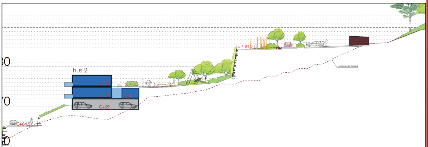
Figur 36. Snitt 2 som viser korleis bustadane er tenkt plassert i terrenget med leik- og uteopphaldsareal mellom (ABO Plan & Arkitektur AS).
