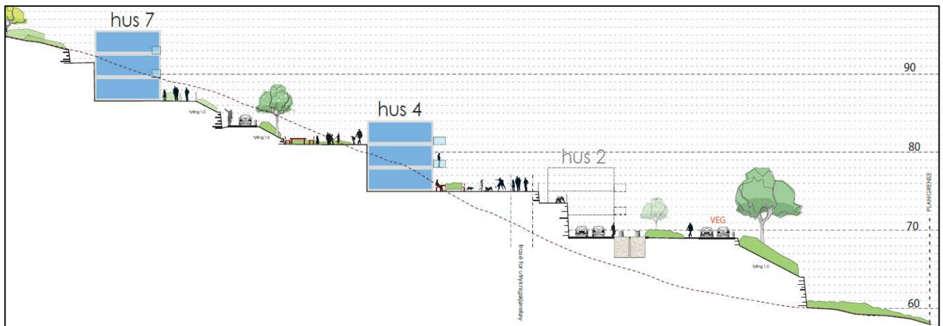
Figur 17. Snitt 2 som viser bygningane innanfor område (BBB1b stipla) BBB4 og BKS6 samt gatetun og leikeområder i terrenget. (ABO Plan & Arkitektur AS).
