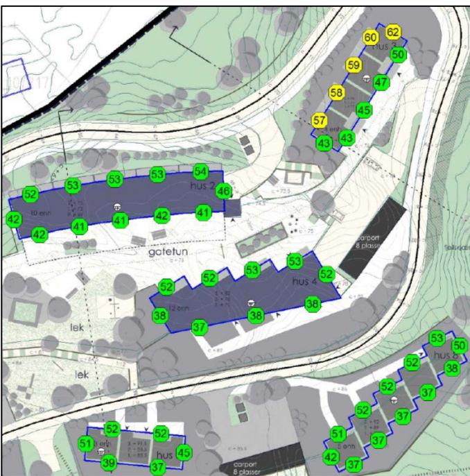
Figur 38. Utsnitt støynivå frå støyrapport (Sweco 18.11.2015).
