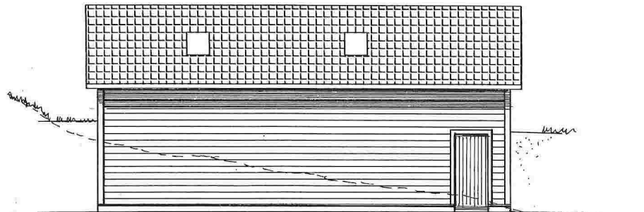
Fasade mot ØST
