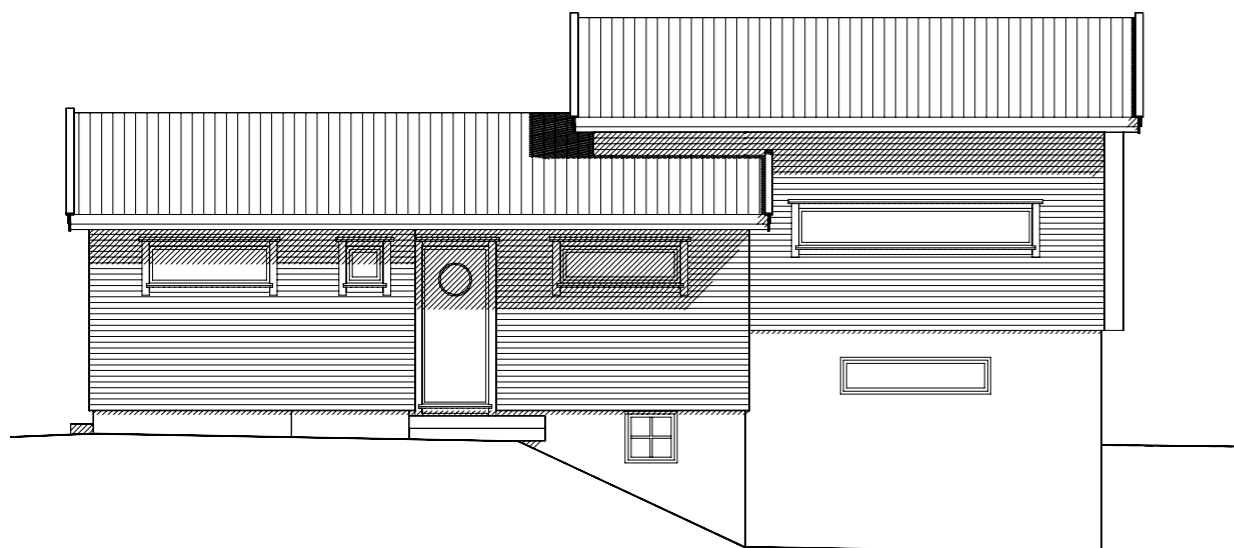
FASADE MOT NORD-ØST Ny situasjon
