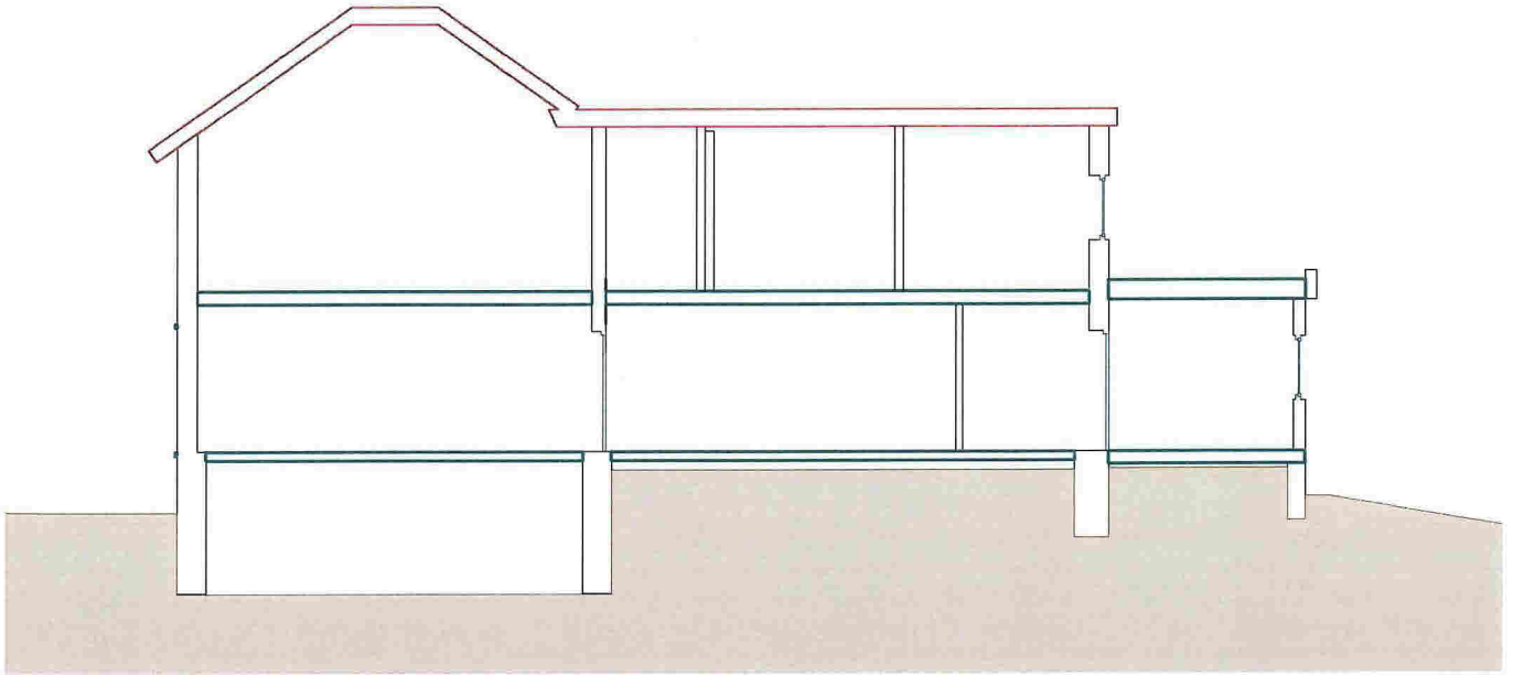
snitt A2 Hovedleilighet-nordfløy) FØR ENDRING
