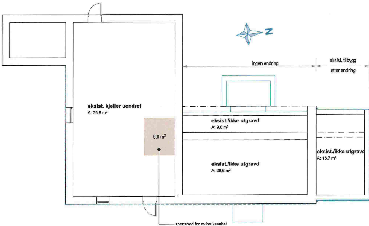
plan kjeller
