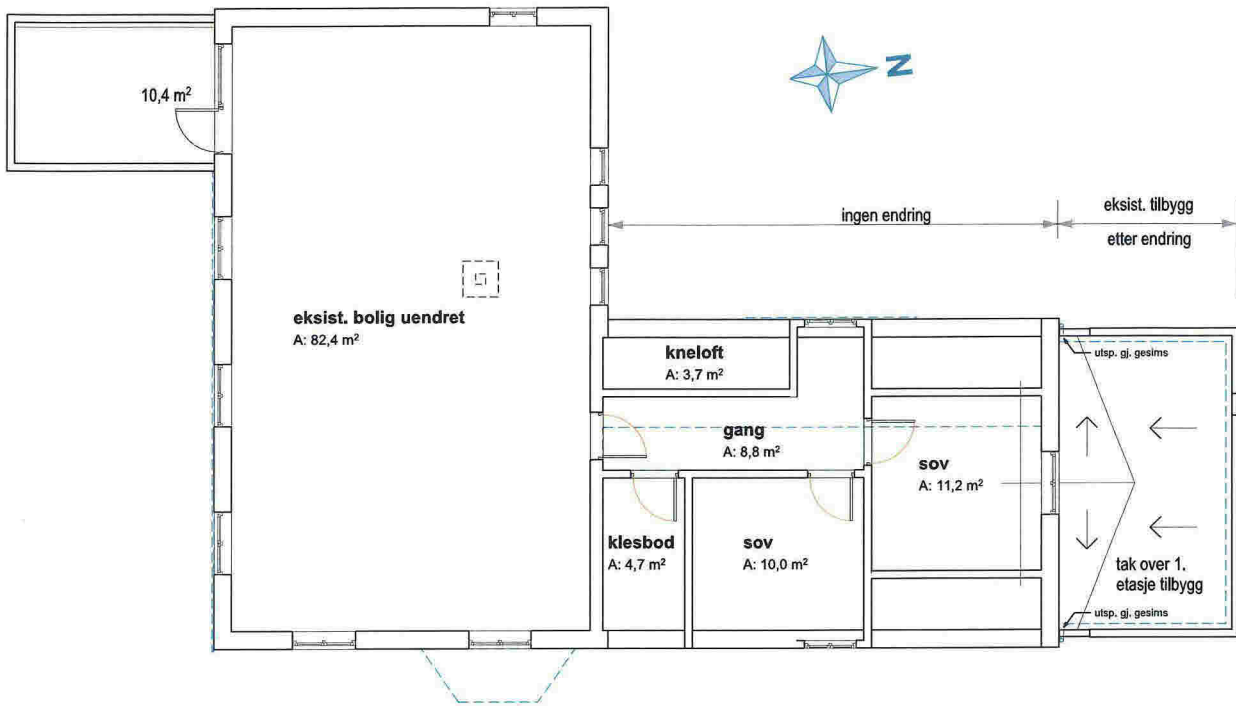
plan 2 etasje
