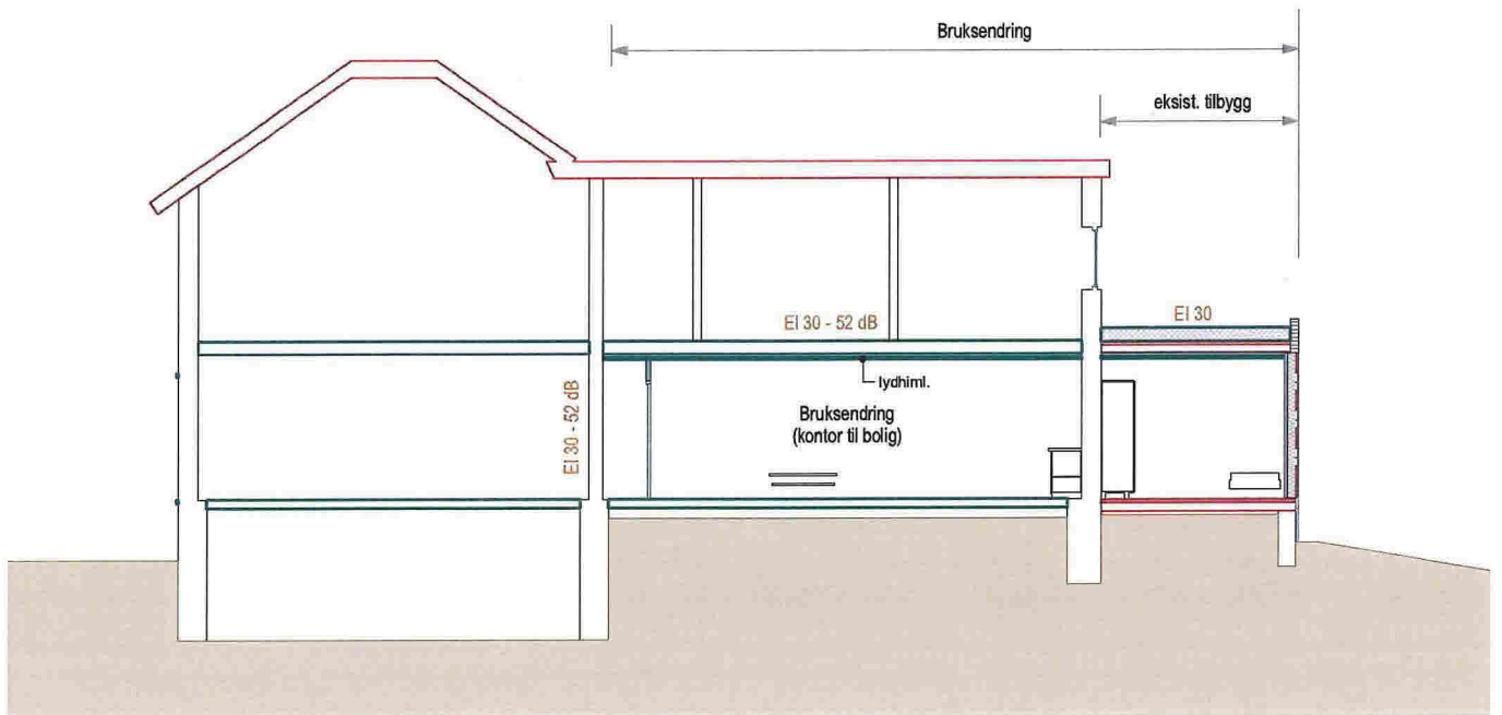
snitt A2 Hovedleilighet-nordfløy) ETTER ENDRING
